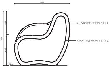
단면도
