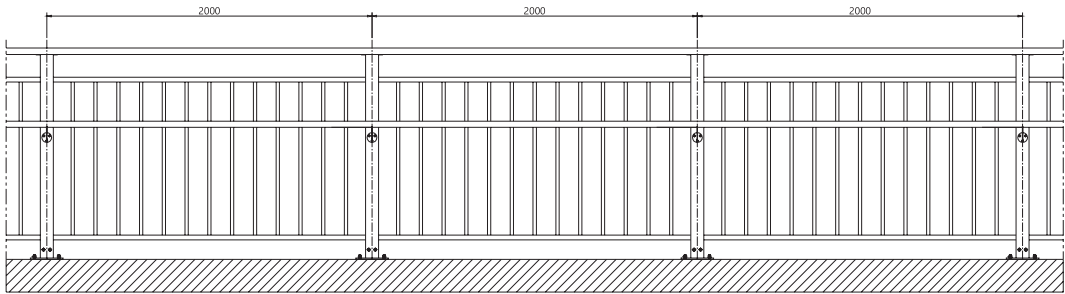
전개도
