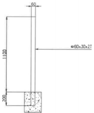
측면도
