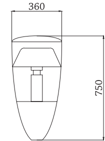
헤드 정면도-1
