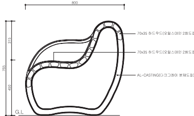
측면도
