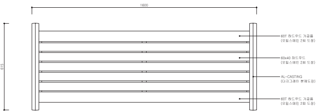
평면도
