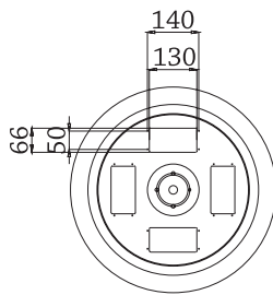
헤드 저면도
