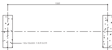
기초 평면도
