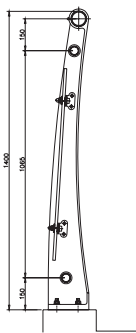
단면도
