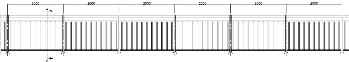
전개도
