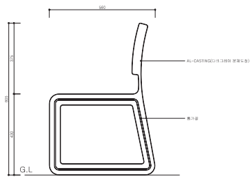
단면도
