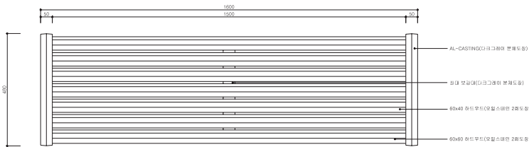
평면도
