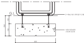
기초 상세도
