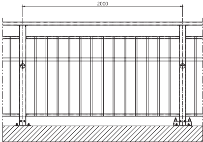
정면도
