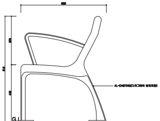
측면도
