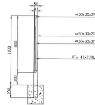
단면도
