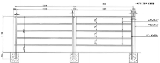
정면상세도
