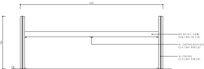
정면도
