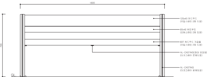
정면도
