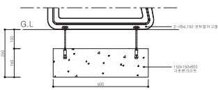
기초 상세도
