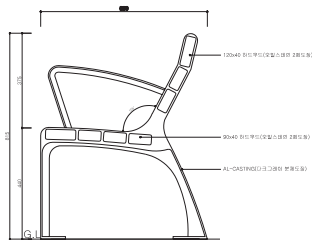
단면도
