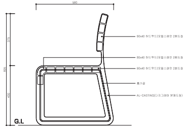
측면도
