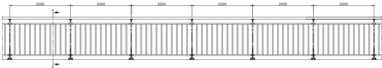
전개도
