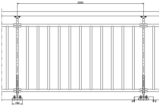
정면도
