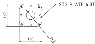
ARM 평면도
