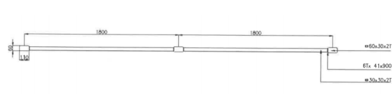
정면도
