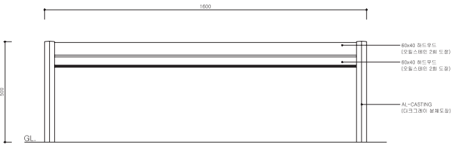
정면도
