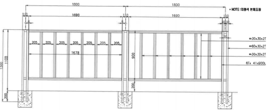
정면상세도
