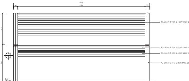
정면도
