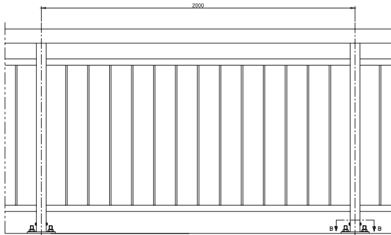
전개도
