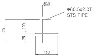
ARM 정면도
