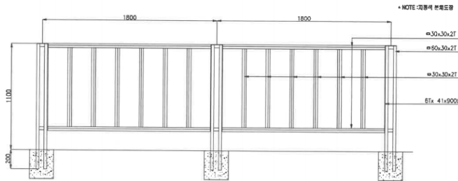
배면도
