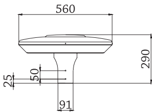
헤드 정면도
