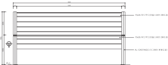
정면도
