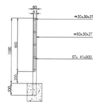
단면도
