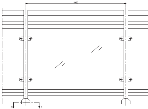
전개도
