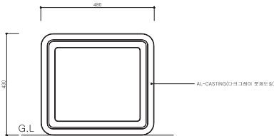
측면도
