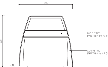
측면도
