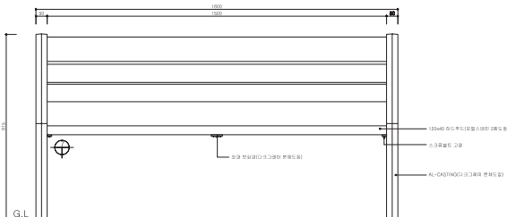
정면도
