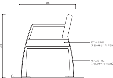
측면도
