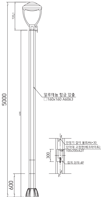
정면도
