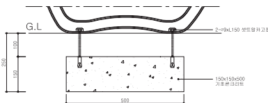
기초 상세도
