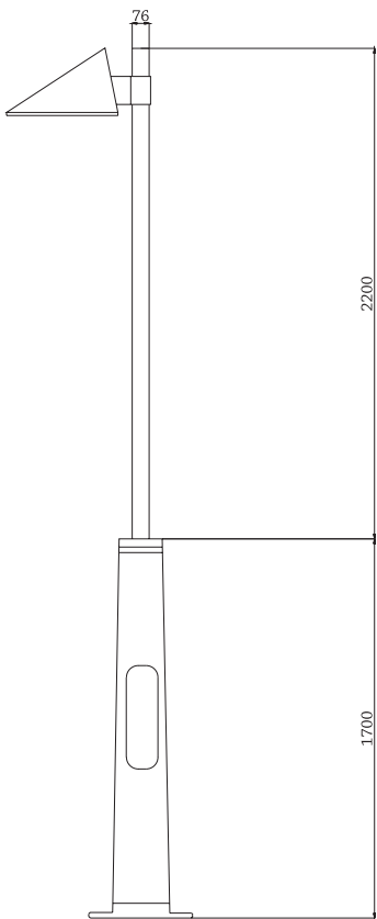
정면도
