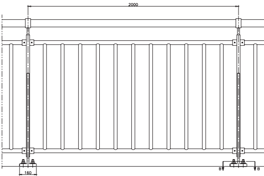
정면도
