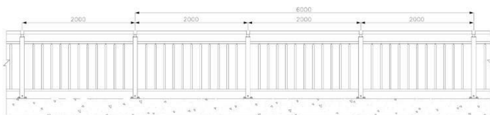
정면도
