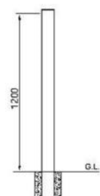
측면도
