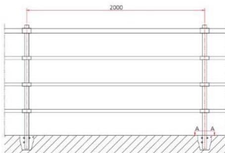
정면도
