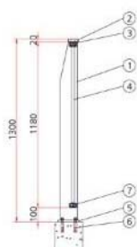
좌측면도
