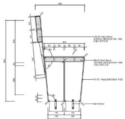
측면도
