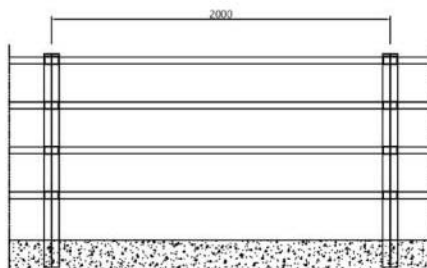
정면도
