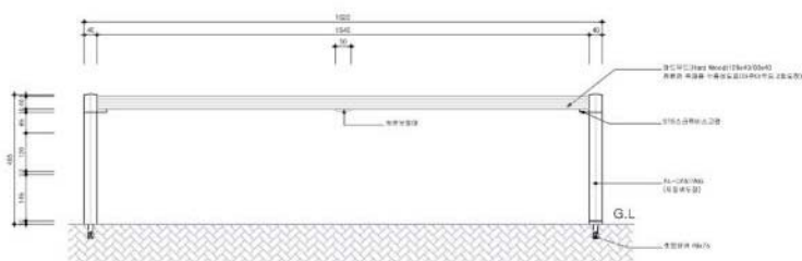
정면도
