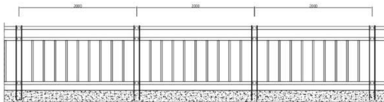
전개도
