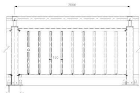
정면 상세도
