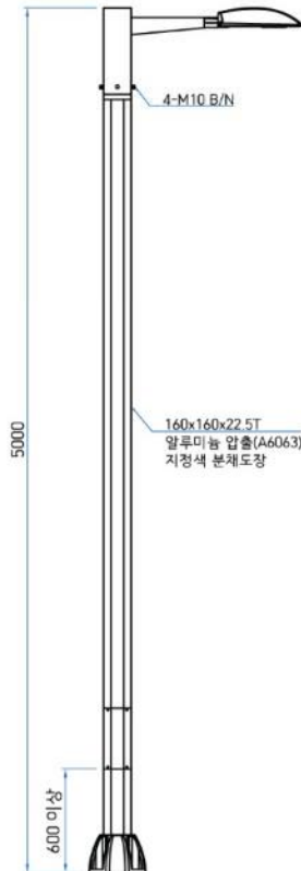
측면도
