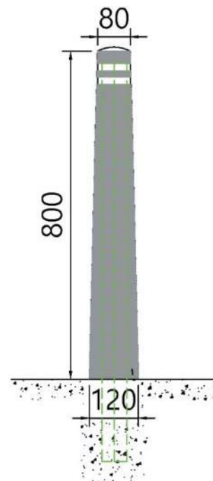
상세도
