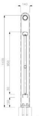
단면 상세도
