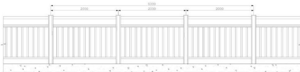
정면도
