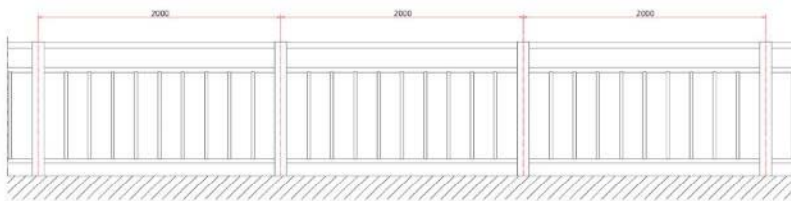
전개도
