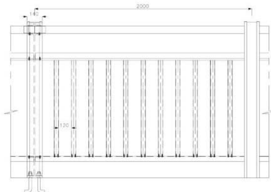
정면 상세도
