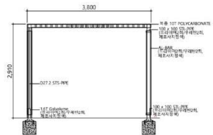
정면도
