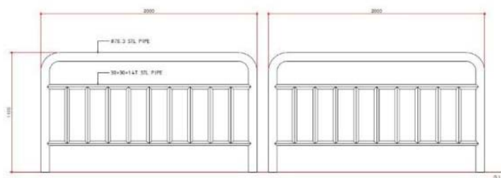
정면도
