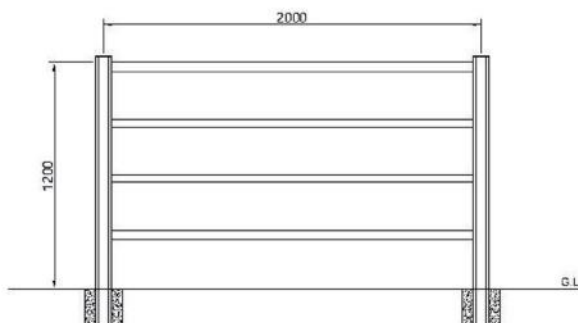
정면도
