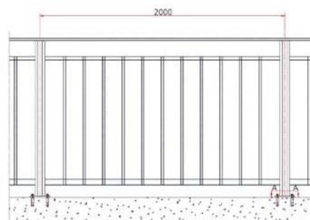
정면도
