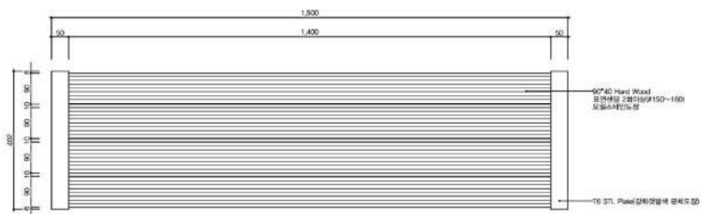
평면도
