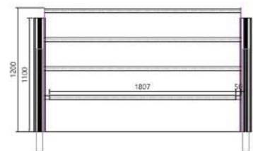
정면 상세도
