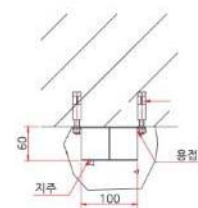
단면도
