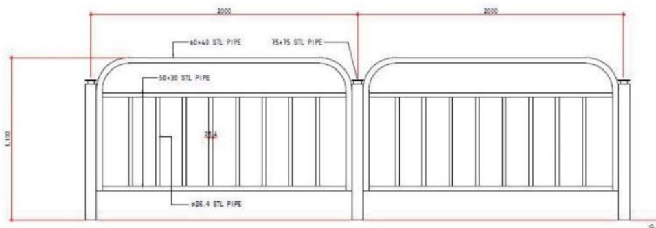
정면도
