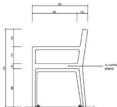
측면도
