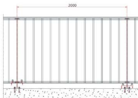
정면도
