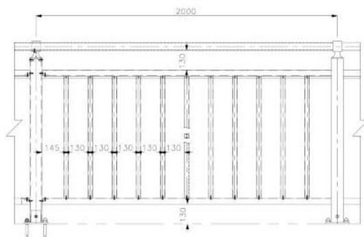
정면 상세도
