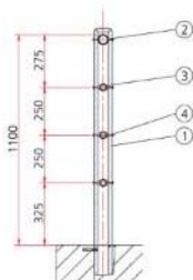
좌측면도
