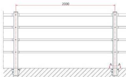
정면도
