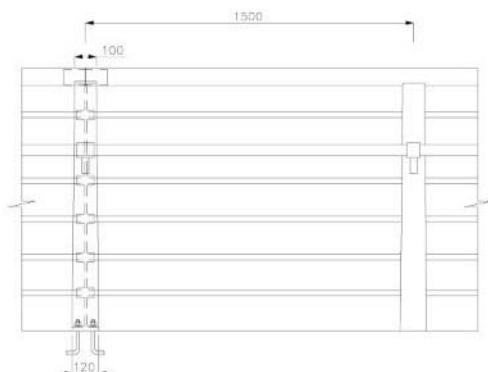
정면 상세도
