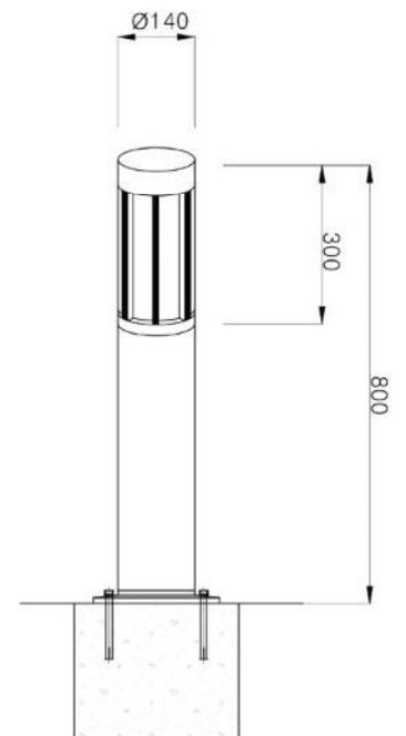
상세도
