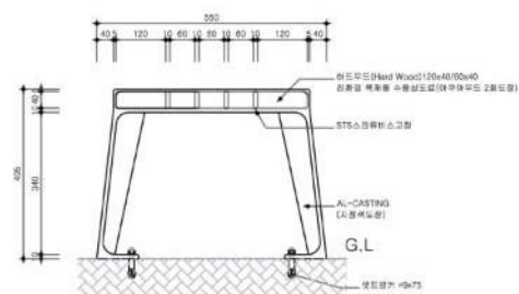
측면도
