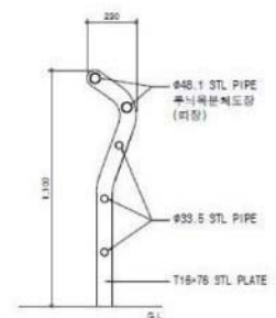
측면도
