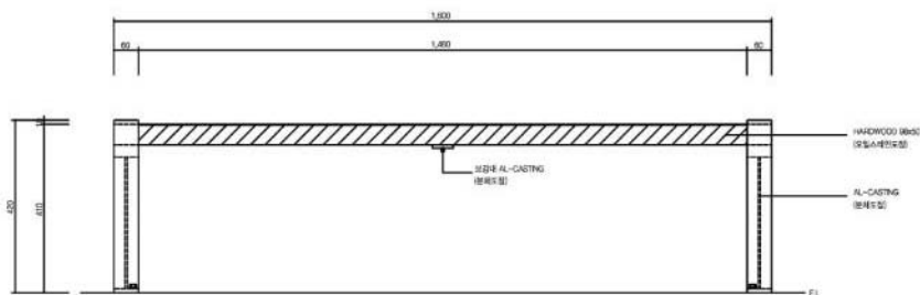
정면도
