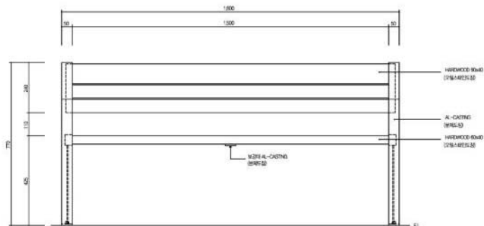
정면도
