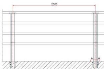
정면도
