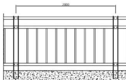
정면도
