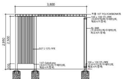
좌측면도
