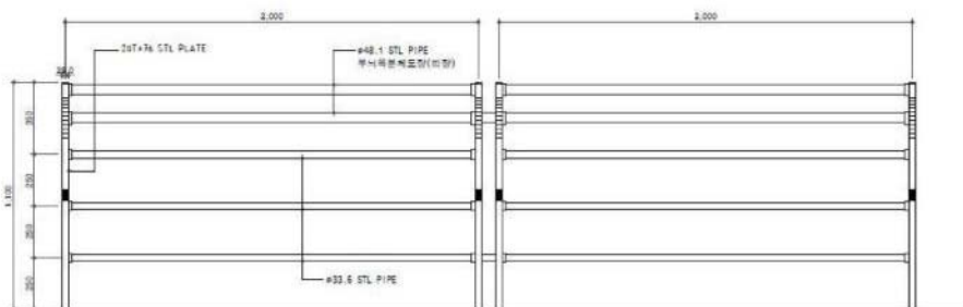
정면도
