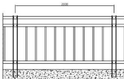
정면도
