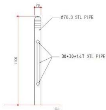
측면도
