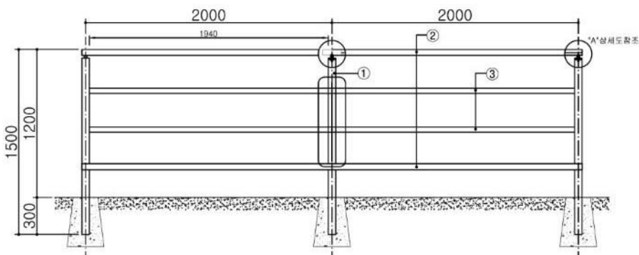
정면 상세도
