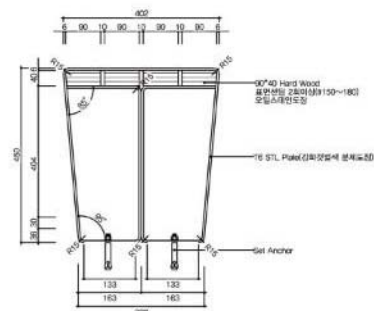
측면도
