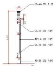
측면도
