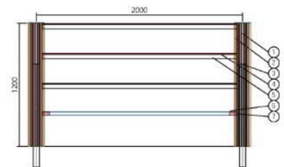
정면 상세도
