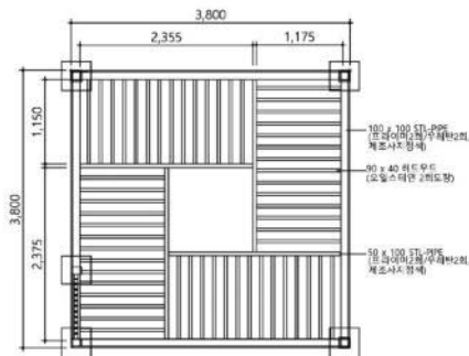
평면도
